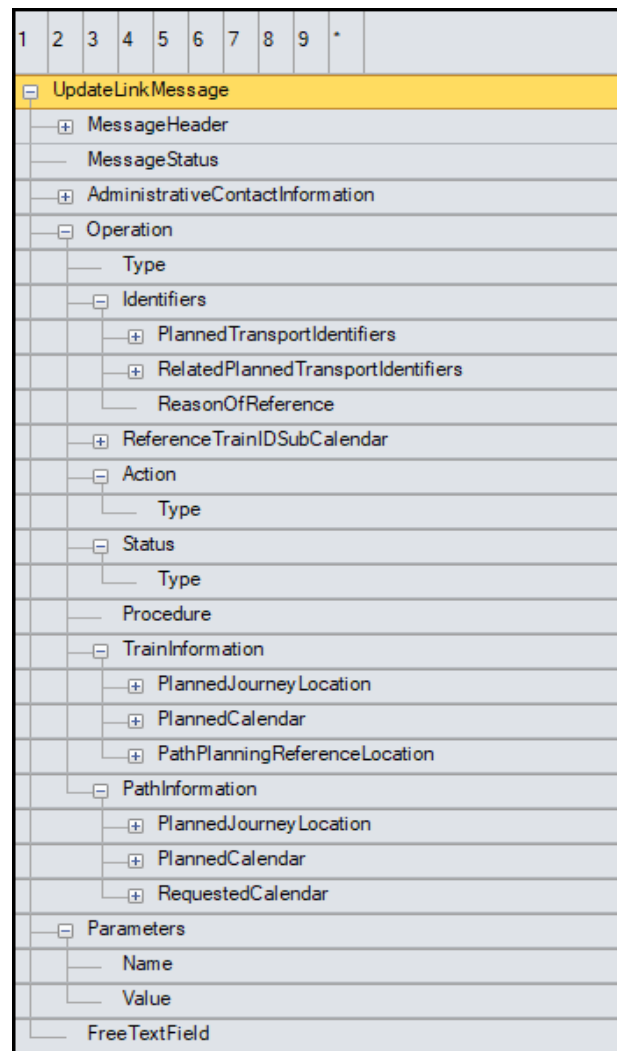
Abbildung 10 UpdateLinkMessage Struktur
