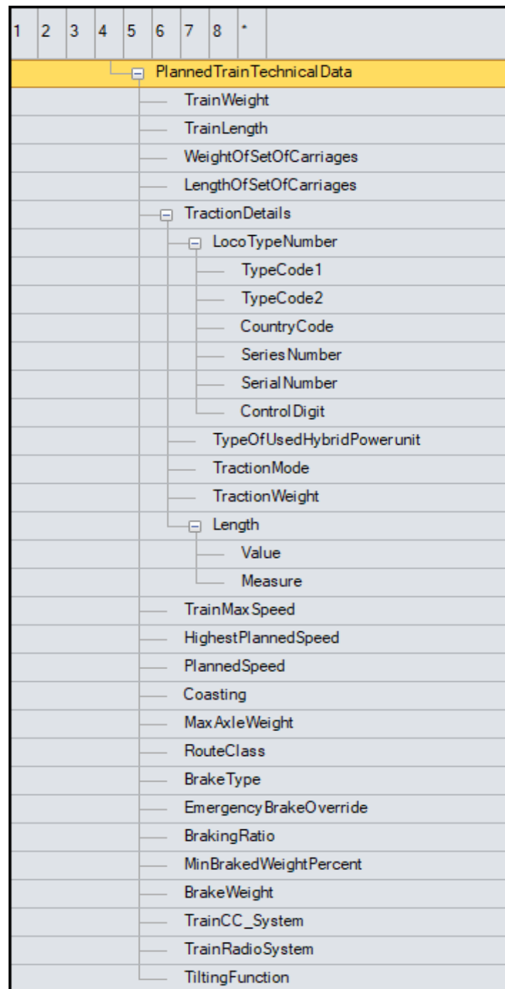
Abbildung 19 PlannedTrainTechnicalData Struktur
