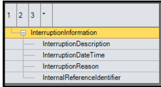
Abbildung 30 InterruptionInformation Struktur
