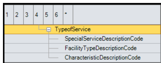
Abbildung 18 TypeOfService Unterstruktur
