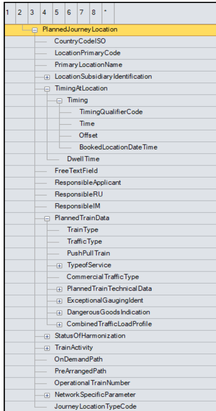
Abbildung 16 PlannedJourneyLocation Strukturübersicht
