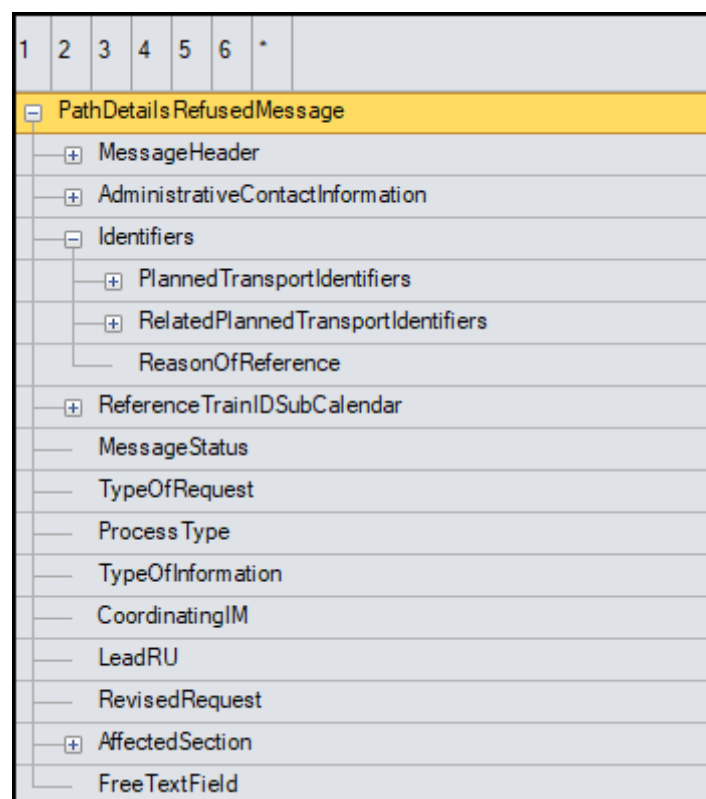
Abbildung 3 PathDetailsRefusedMessage Hauptstruktur
