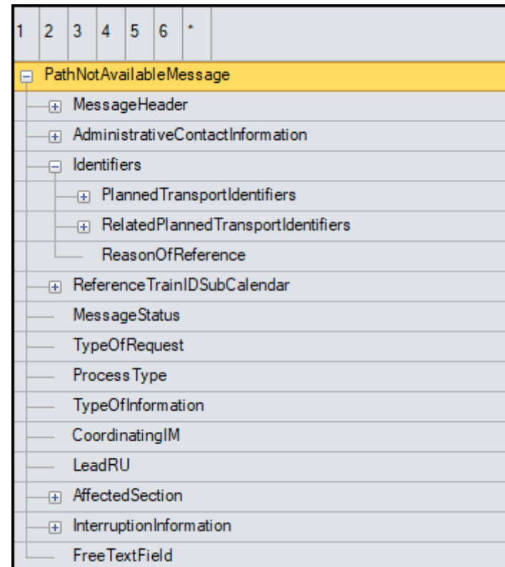
Abbildung 6 PathNotAvailableMessage Hauptstruktur
