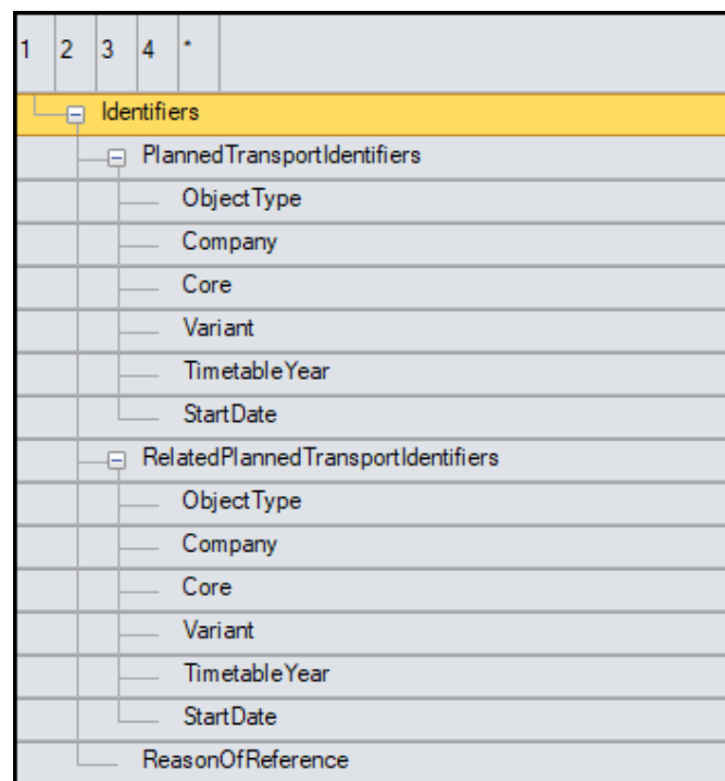
Abbildung 13 Identifiers Struktur
