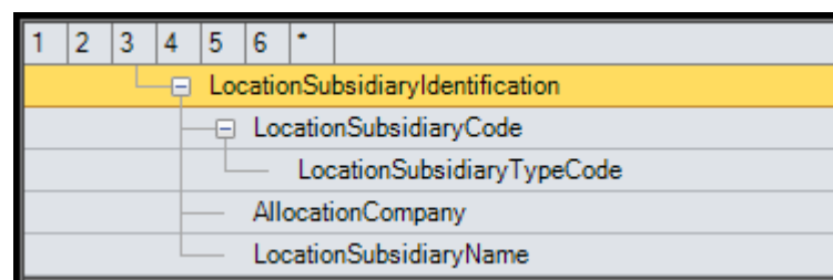
Abbildung 17 LocationSubsidiaryIdentification Unterstruktur
