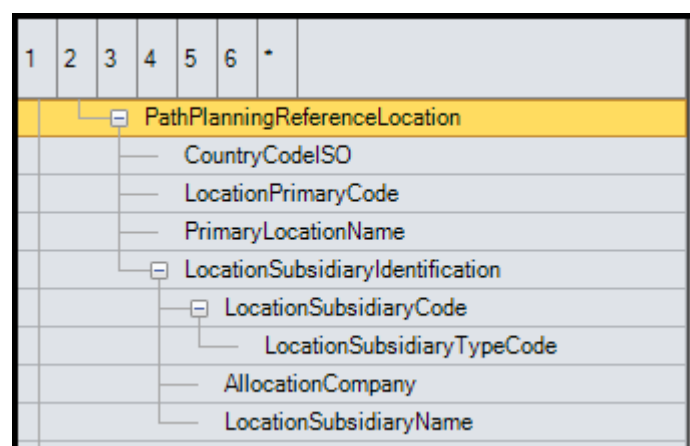
Abbildung 28 PathPlanningReferenceLocation Struktur
