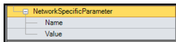
Abbildung 31 NetworkSpecificParameter Struktur
