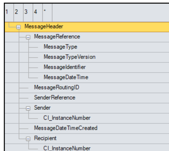
Abbildung 11 MessageHeader Struktur
