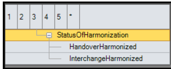
Abbildung 23 StatusOfHarmonization Unterstruktur
