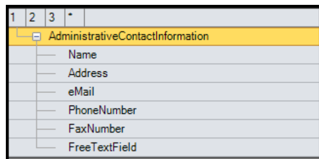
Abbildung 12 AdministrativeContactInformation Struktur
