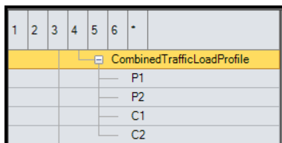
Abbildung 22 CombinedTrafficLoadProfile Unterstruktur
