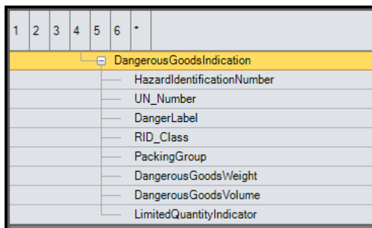
Abbildung 21 DangerousGoodsIndication Unterstruktur
