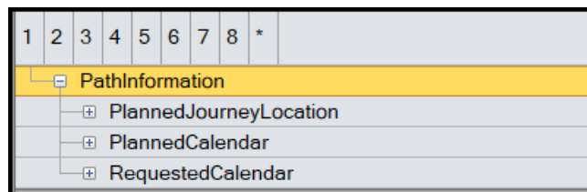
Abbildung 15 PathInformation Oberstruktur
