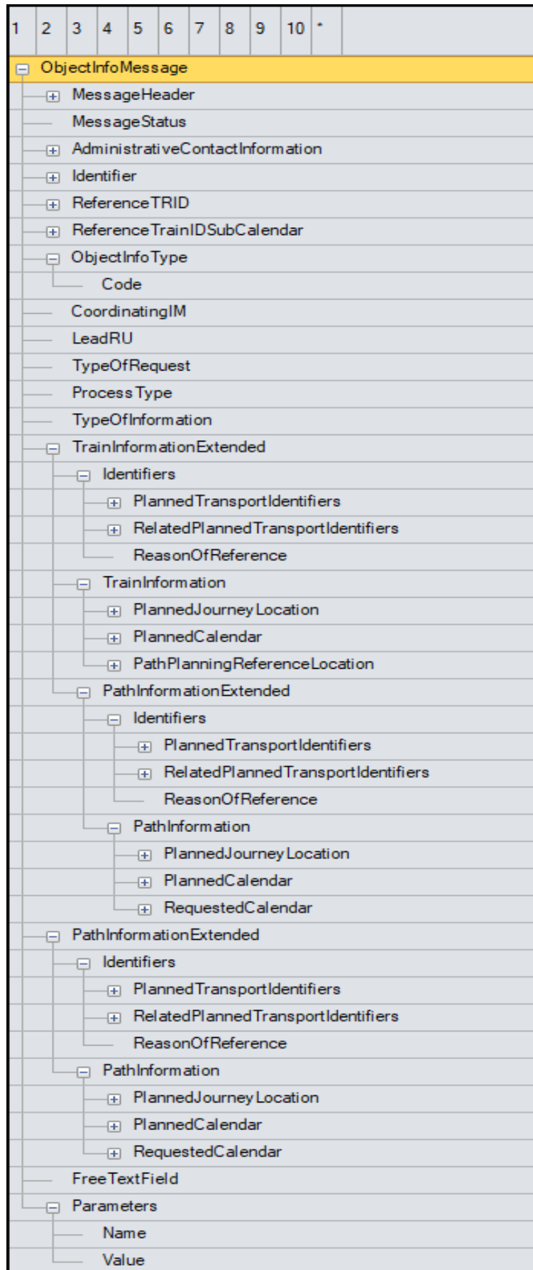
Abbildung 9 ObjectInfoMessage Struktur
