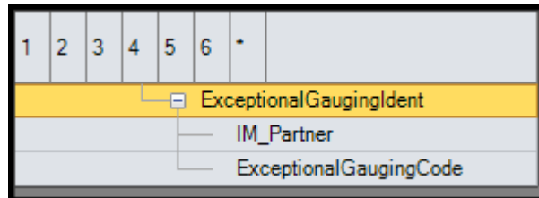
Abbildung 20 ExceptionalGaugingIdent Unterstruktur
