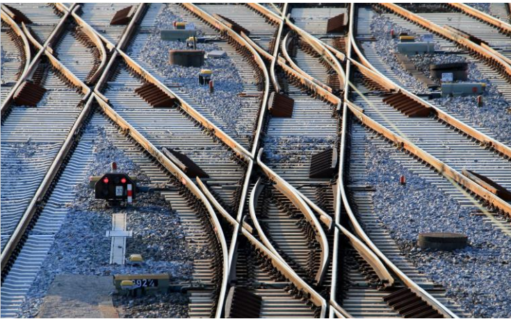
Weichen und Gleisverbindungen im Nürnberger Rbf, DB AG/Uwe Miethe
